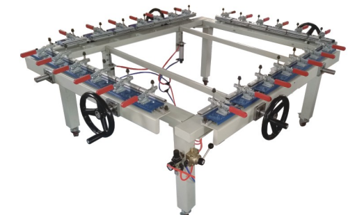
机械式链条绷网机(半气动)
